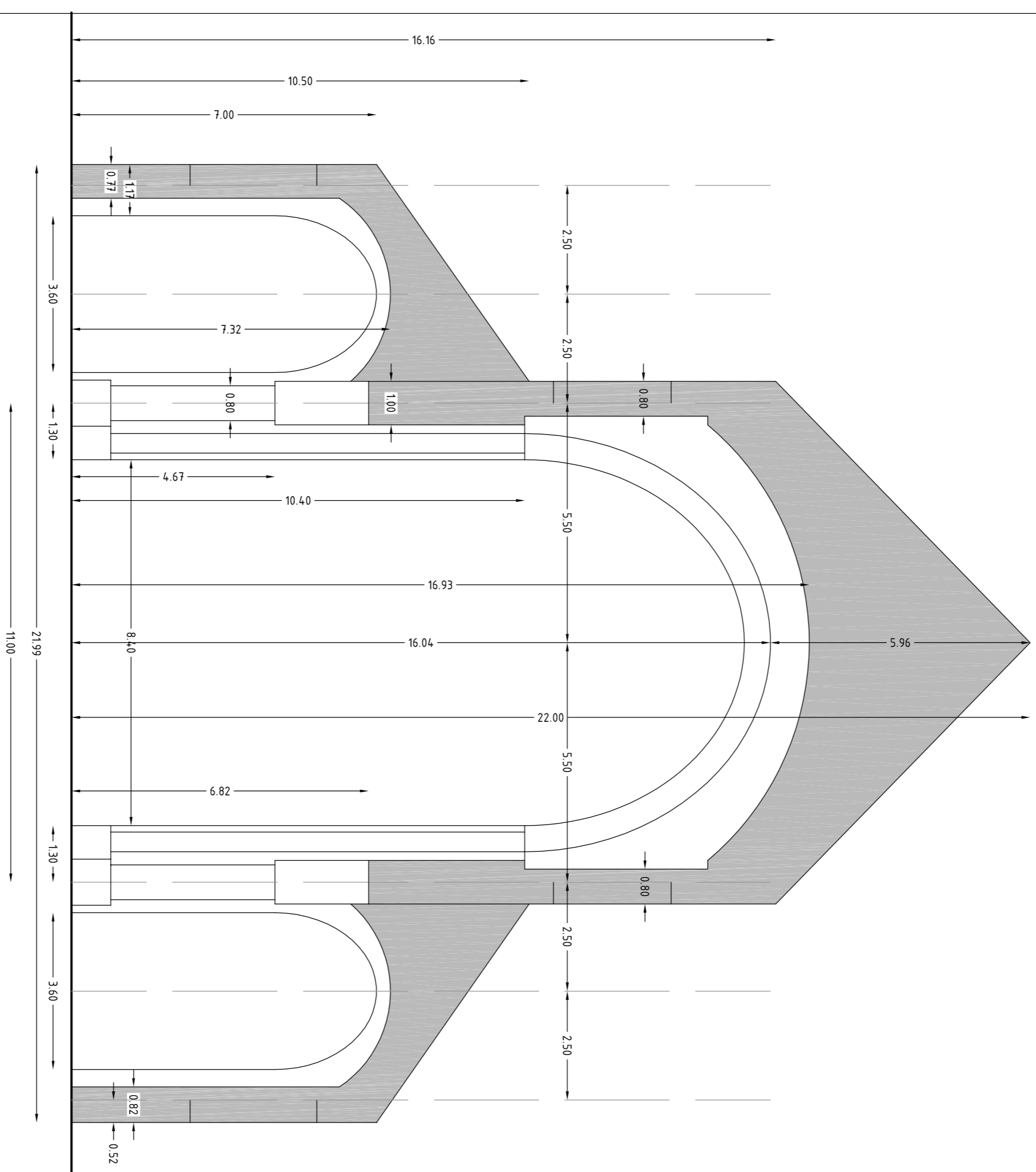
DWARSDOORSNEDE - SCHAAL: 1/100
