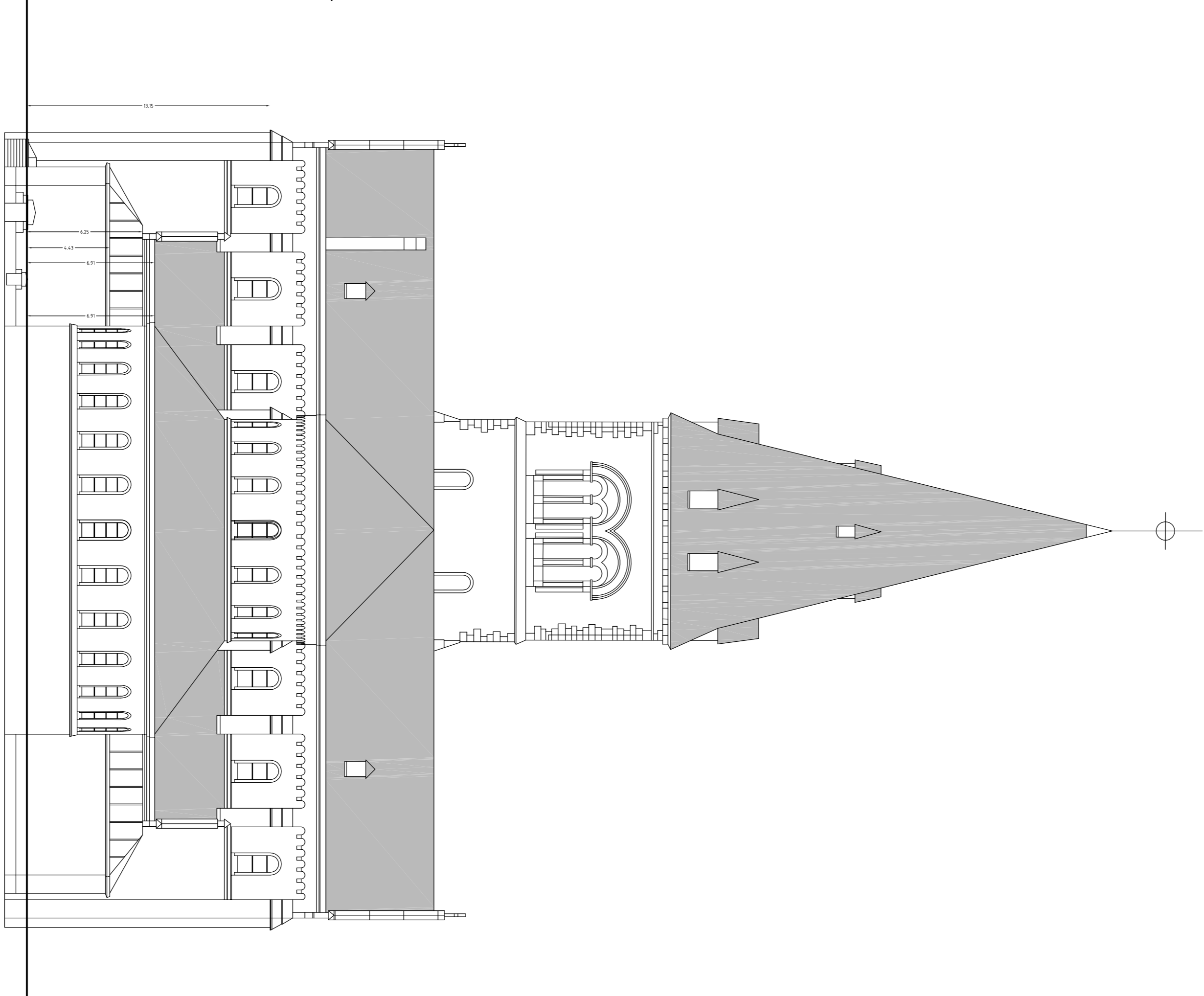
GEVEL WEST
